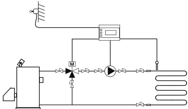
Εικόνα 3 Εφαρμογή αντιστάθμισης με τρίοδη αναμεικτική βάνα
