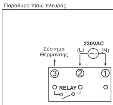
Εικόνα 1 Κλέμα ηλεκτρολογικής σύνδεσης
